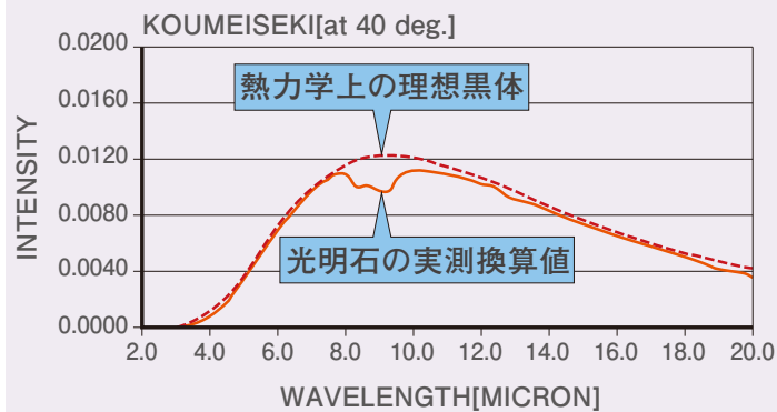
光明石の遠赤外線放射データ
